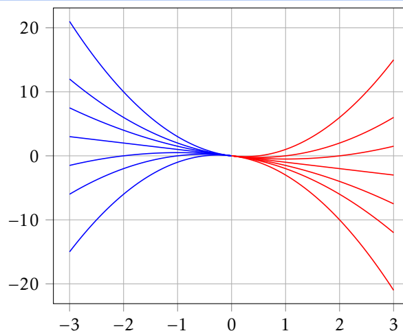
FIGURE 1 – Tracé de quelques solutions de l'équation différentielle tx' - 2x = t .
