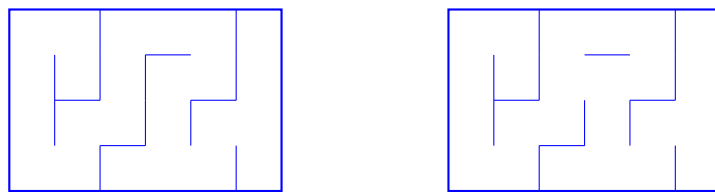
FIGURE 2 – À gauche, un labyrinthe parfait ; à droite un labyrinthe imparfait.
